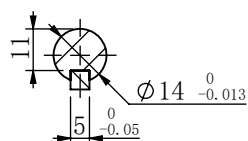
剖面 A-A
