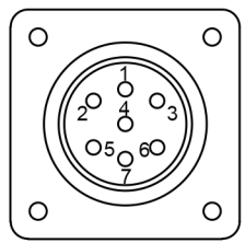
绝对值编码器插头(Q向)
