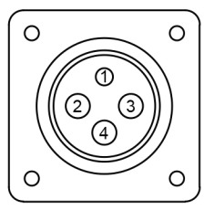
动力线航空插头(P向)
