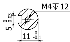
剖面 A-A
